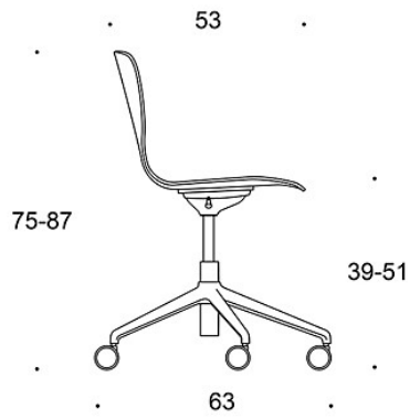
377RGS (RGSC/RGSBC/RGSD)
